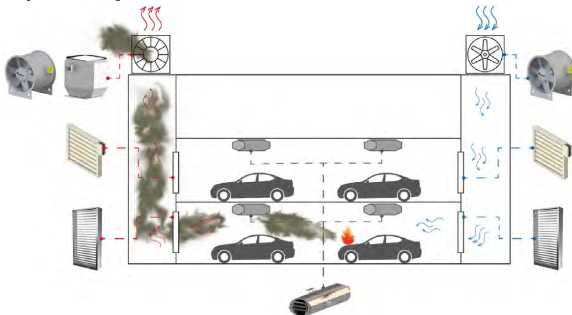
Rys. 4 Schemat garażu.
